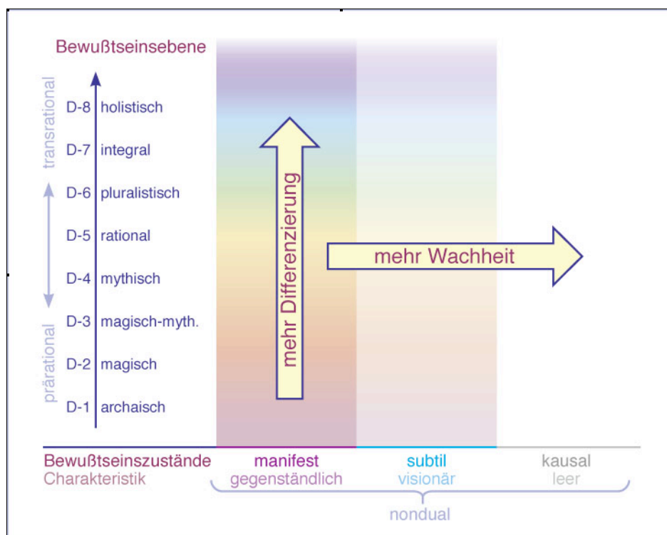
Abb. 1: Die Wilber-Combs-Matrix
